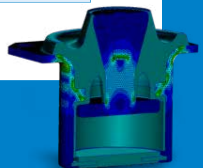
Diseño final
