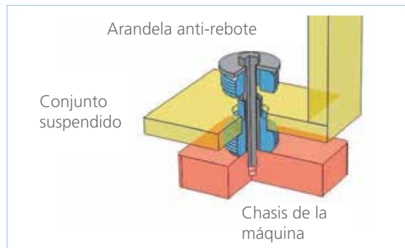
- MONTAJE 2
