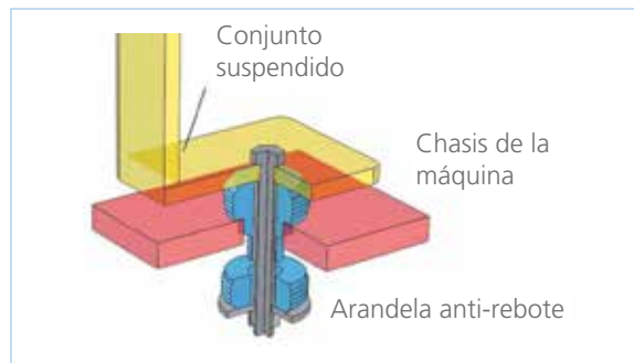
- MONTAJE 2
