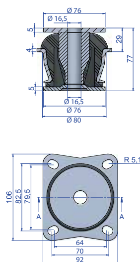
Arandela superior Cono 30 código 608074 Arandela inferior Cono 30 código 608125
