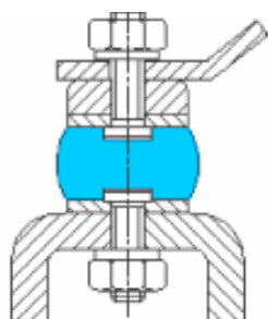
Compresión
