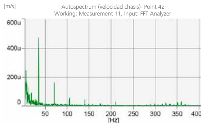
Chasis FFT
