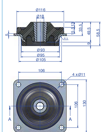
Arandela superior Cono 141 código 610285 Arandela inferior Cono 141 código 606766
