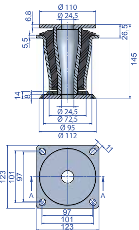
Arandela superior Cono 70 código 608033 Arandela inferior Cono 70 código 606145
