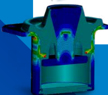
Diseño inicial
