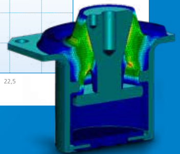
Simulación FEM
