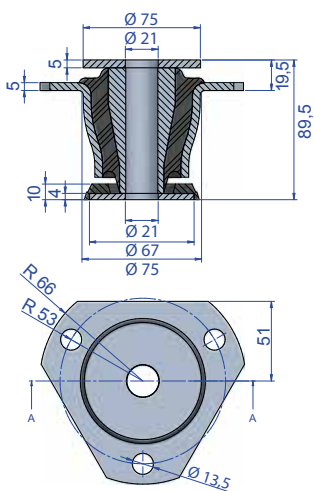
Arandela superior Cono 40 código 610027 Arandela inferior Cono 40 código 608267
