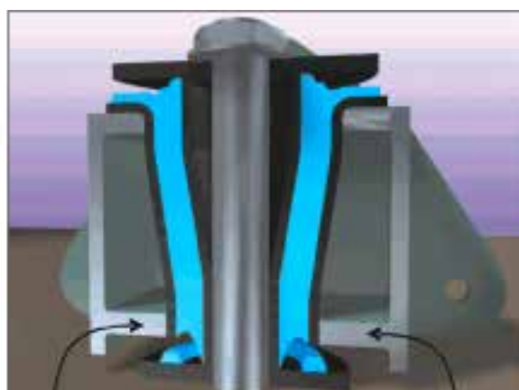
Restringidores de carga radial
