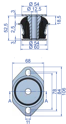
Arandela superior Cono 12 código 611068 Arandela inferior Cono 12 código 611068
