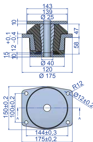
Arandela superior Cono 121 código 606378 Arandela inferior Cono 121 código 606379
