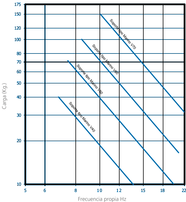
FRECUENCIA PROPIA AMC MECANOCAUCHO® TIPO MARINO EN V
