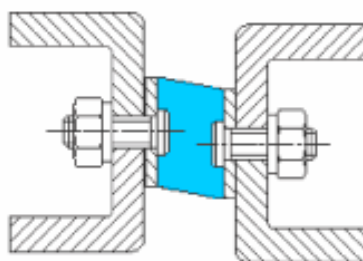
Cizalladura
