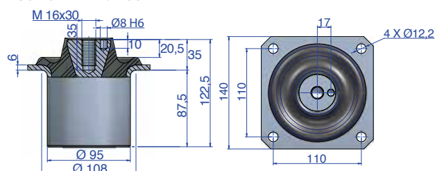
CONO HIDRÁULICO 72
