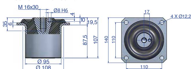
CONO HIDRÁULICO 71
